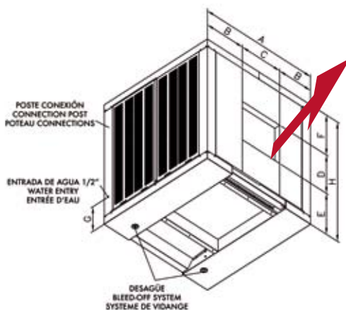
FILTRO DE VIRUTA DE MADERA WOOD FIBER FILTER FILTRE DE FIBRE DE BOIS
