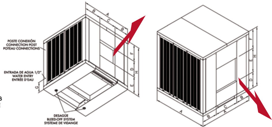
FILTRO DE CELULOSA. NIDO DE ABEJA CELLULOSE COOLING PAD. HONEYCOMB PANNEAU DE CELLULOSE. NID D'ABEILLE mm=100
